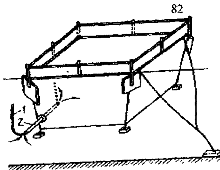
Рис. 12. Личинковий садок 1 – повітропровід. 2 – ерліфтне пристосування
