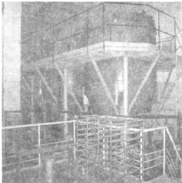
Рис. 35. Біологічний фільтр установки замкнутого водопостачання
