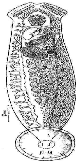
Рис. 53. Схеми будови Nitzschia sturionis
