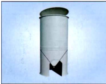
Круглий циркуляційний басейн конічної форми, на ніжках з шаровим краном із ПВХ, ухилом дна 45^{\circ}
