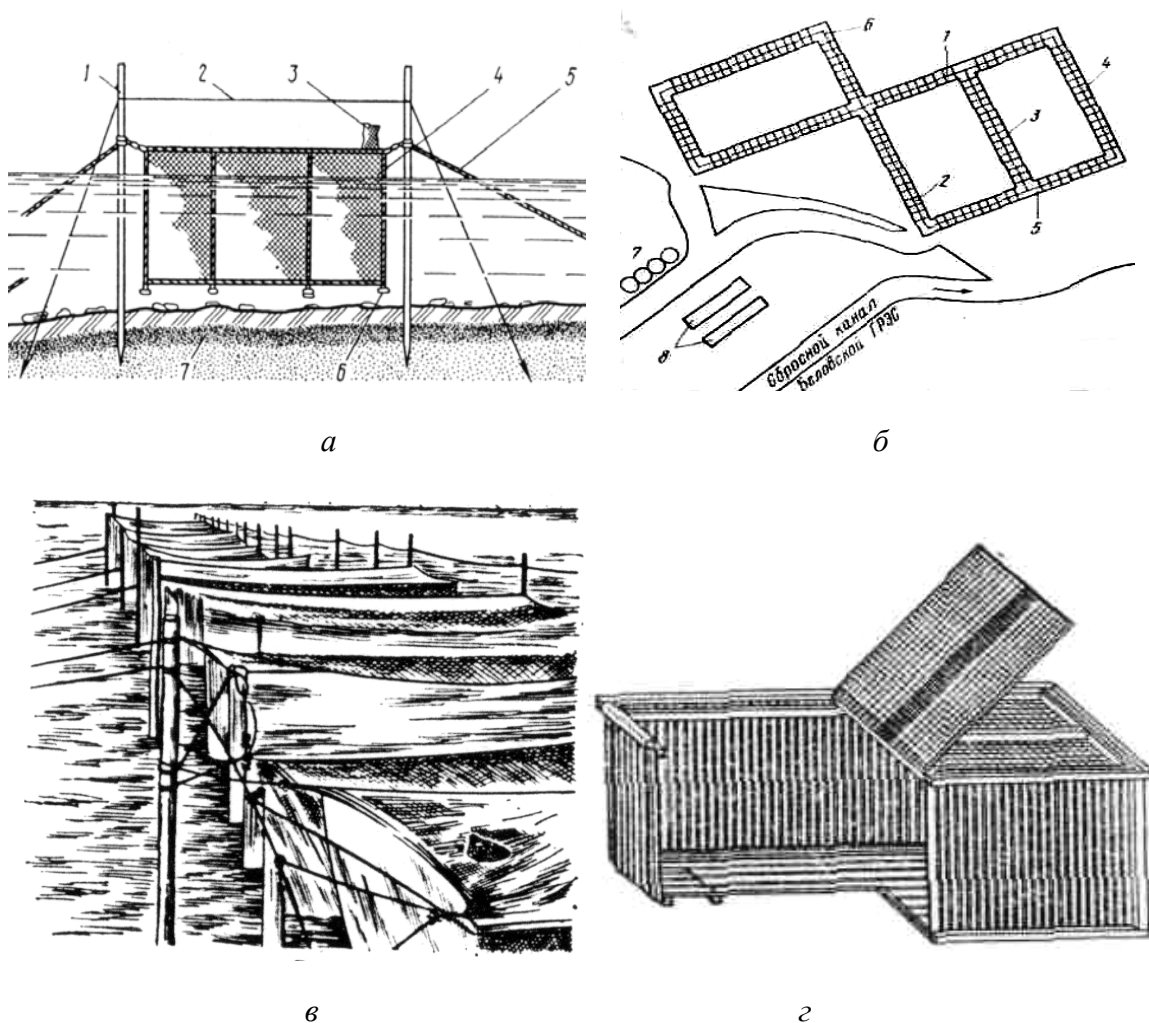
Рис. 21. Стационарные садки: а – конструкция садка: 1 – гундеры; 2 – проволоочная рама; 3 – сетчатый рукав для посадки в садок рыбы и раздачи корма; 4 – садок; 5 – трос, крепящий гундеры; 6 – грузы; 7 – грунт; б – общий вид; в – стационарный настил на водоеме-охладителе Беловской ГРЭС; г – садок из реек
