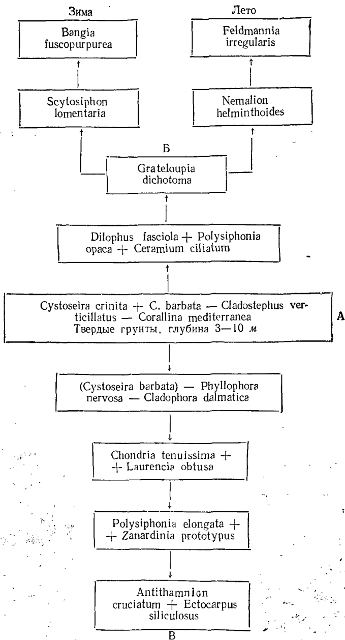
Схема эколого-фитоценологических рядов вертикального распределения ассоциаций у открытых берегов Черного моря. Ряд А — Б: уменьшение глубины, увеличение прибойности; ряд А — В: увеличение глубины, уменьшение прибойности.
