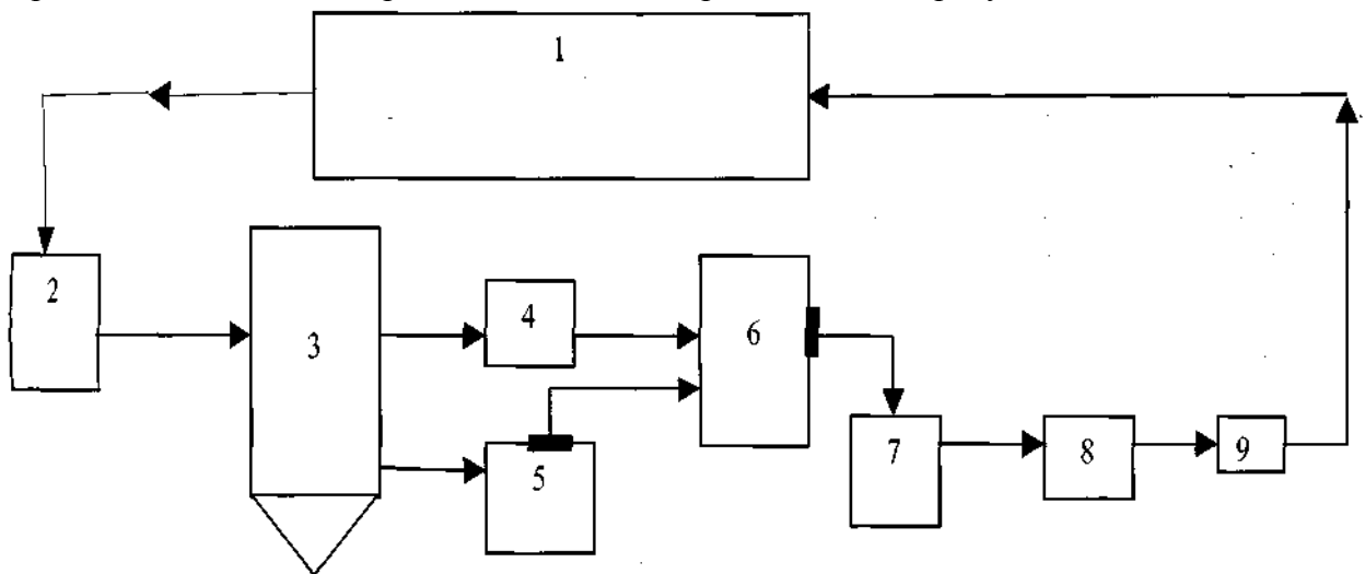
Рис. 31. Принципиальная схема установки 1 - рыбоводные емкости; 2 — фильтр грубой очистки; 3 — блок биологической очистки; 4 - блок регулировки pH; 5 — фильтр тонкой механической очистки; 6 — блок терморегуляции; 7 — бактерицидная установка; 8 — аэрактор; 9 — озонатор
