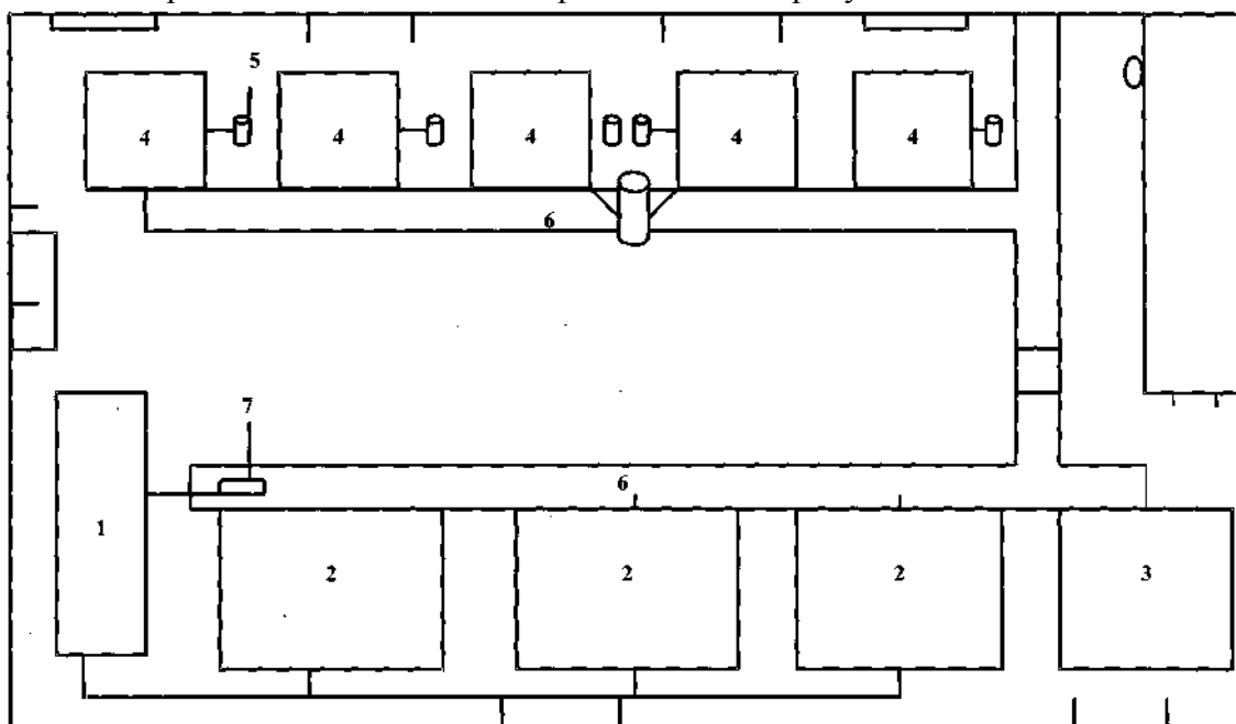
Рис. 26. Схема рыбоводного комплекса научно-экспериментальной базы «Кагальник» 1 — биофильтр; 2 — бассейны 2x2x0,7 м; 3 — отстойник; 4 — бассейны 1x1x0,5; 5 — фильтр Hydor; 6 — сливной желоб; 7 — погружной насос
