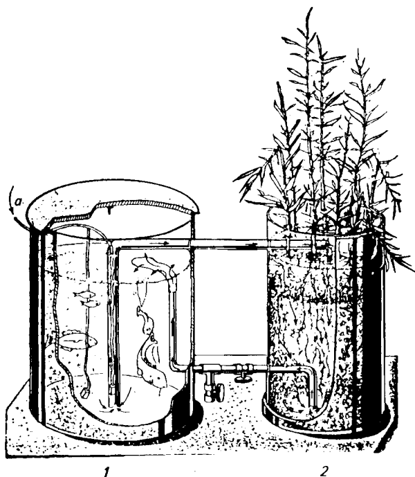
Рис. 42. Замкнутая система для полунтенсивного выращивания рыбы:
