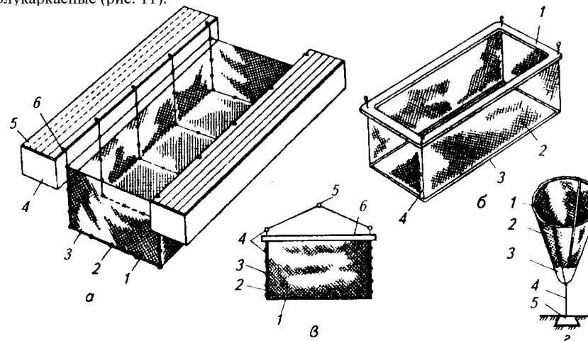
Рис. 11. Садки:
