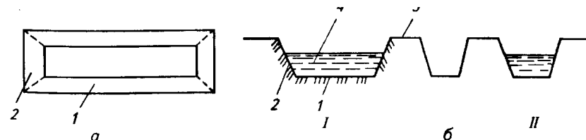
Рис. 1. Копанный (I) и обвалованный (II) пруды:
