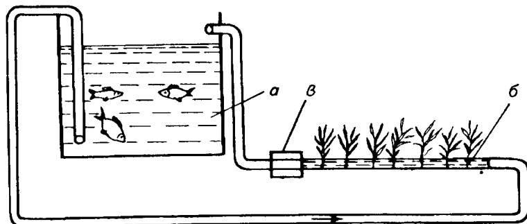
Рис. 43. Гидропонная установка рыба — овощи:
