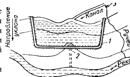
Рис. 2. Ручевой пруд:
