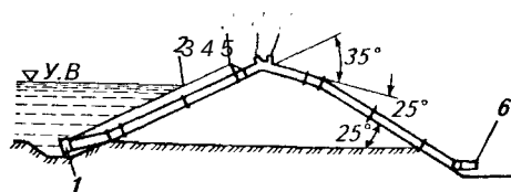
Рис. 7. Сифонный водоспуск:
