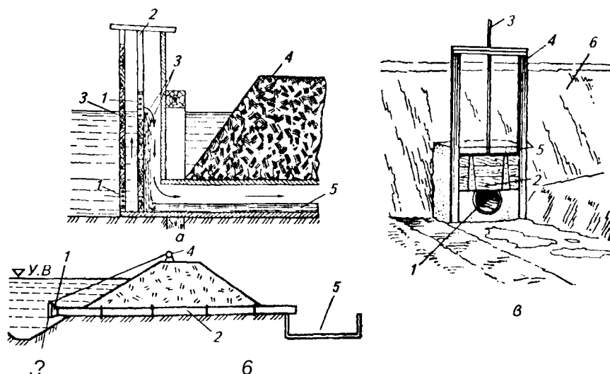
Рис. 6. Донные водоспуски:
