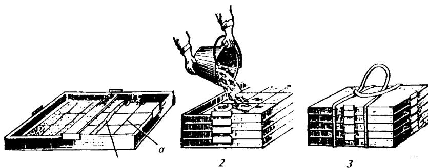
a — сетка-каркас; б — карманы; 1 — ящик для транспортирования; 2 — укладка посадочного материала; 3 — стопка ящиков
